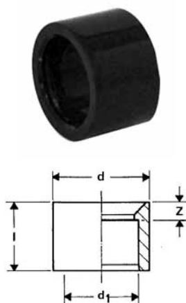
Redukcia na lepenie
