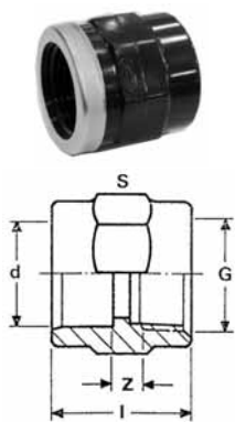
Mufňa na lepenie x závit s výstužným krúžkom, PN 16
