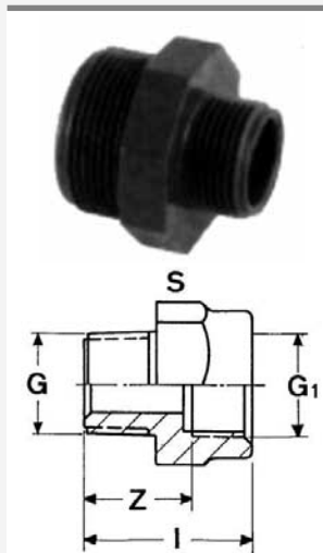
Závitová redukcia vonkajší závit x vonkajší závit, PN 16
