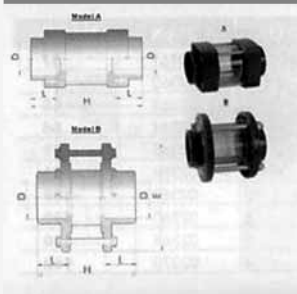
Priezor na kontrolu kvapalín (na lepenie)
