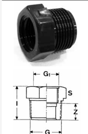
Redukcia krátka vonkajší závit x vnútorný závit, PN 16
