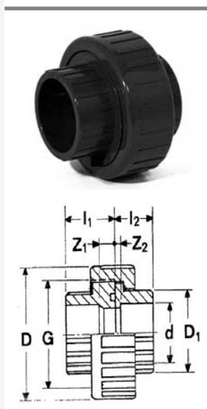
Šrobenie na lepenie, PN 16
